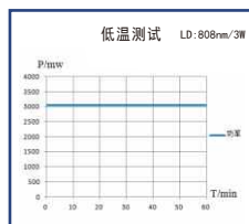
25°C功率曲线
